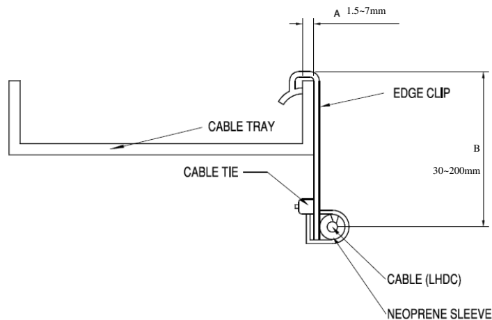
Figure 8.3 – Edge clip
